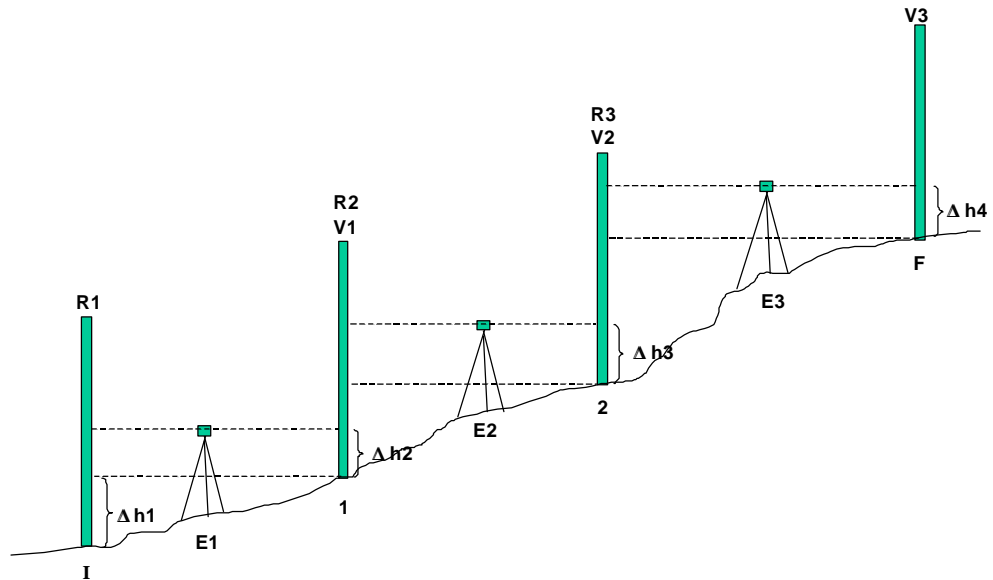
Figura 172 – Nivelamento Linear Composto
