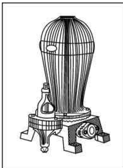
Figura 72 - Carneiro Hidráulico
