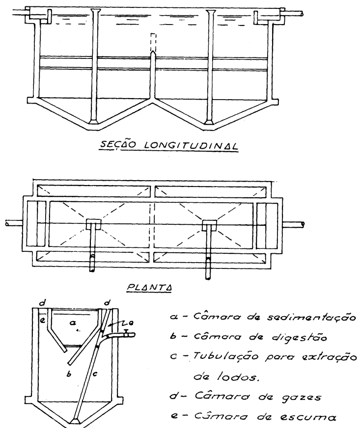
Figura 112 - Tanque Imhoff
